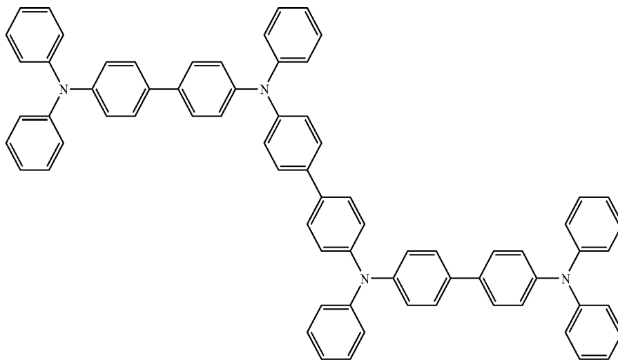
TPTE1
