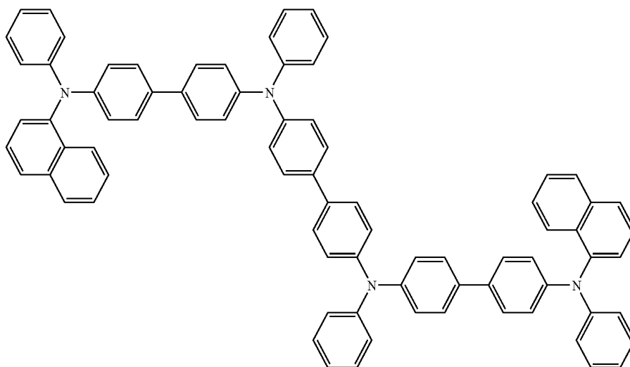
NTPA
