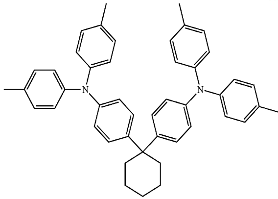
HTM2
