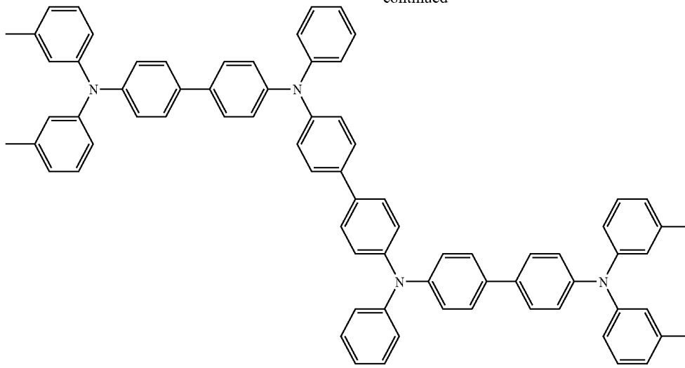
TPTE2
